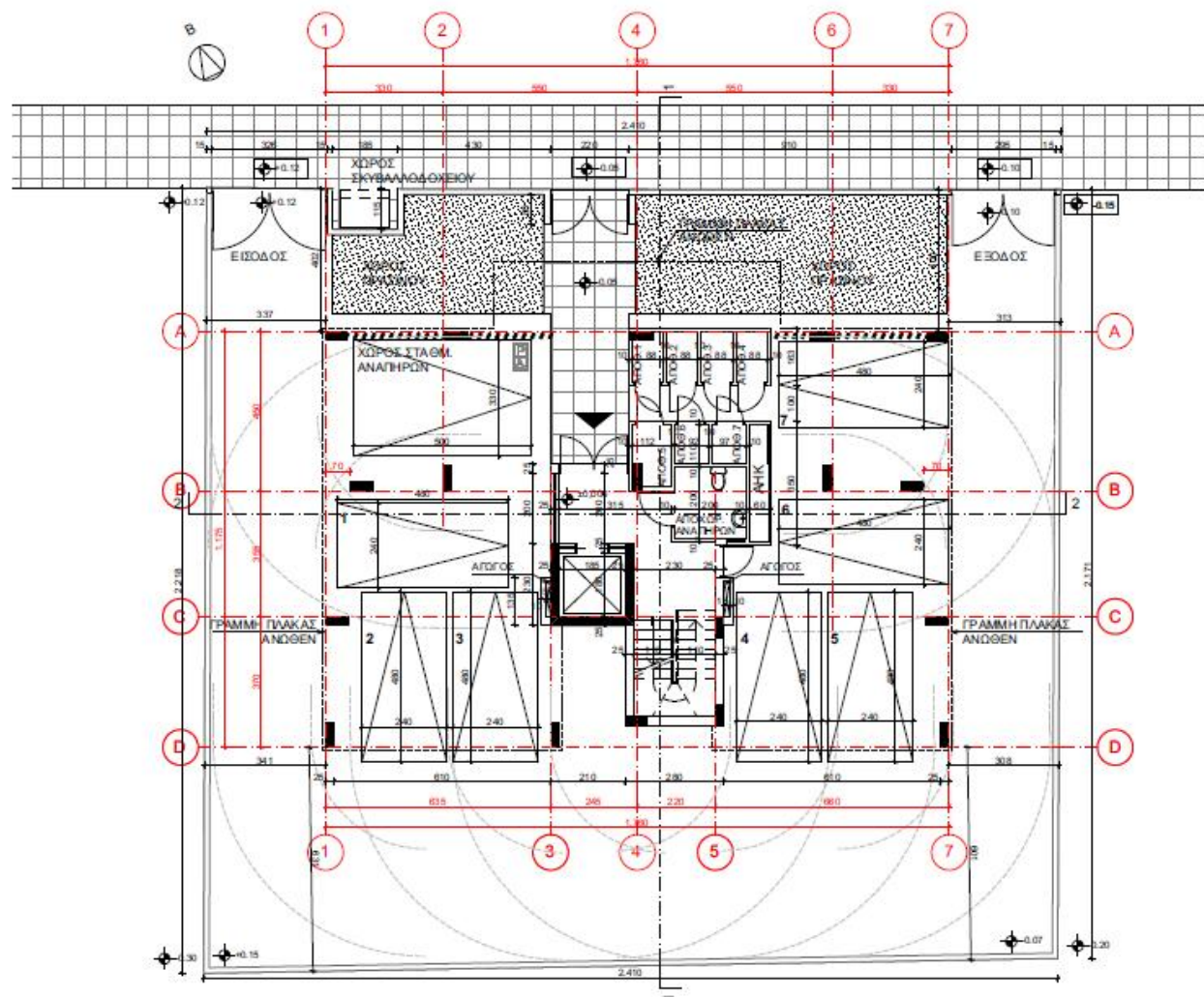
ΚΑΤΩΦΗ ΣΟΓΕΙΟΥ
