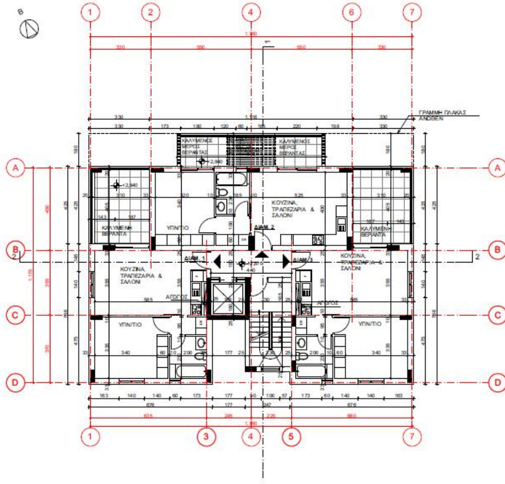
ΚΑΤΩΦΗ Α ΟΡΟΦΟΥ
