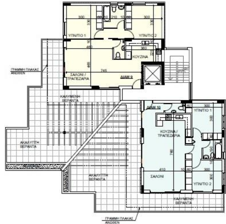
ΚΑΤΟΠΗ 'Β ΟΡΟΦΟΥ
