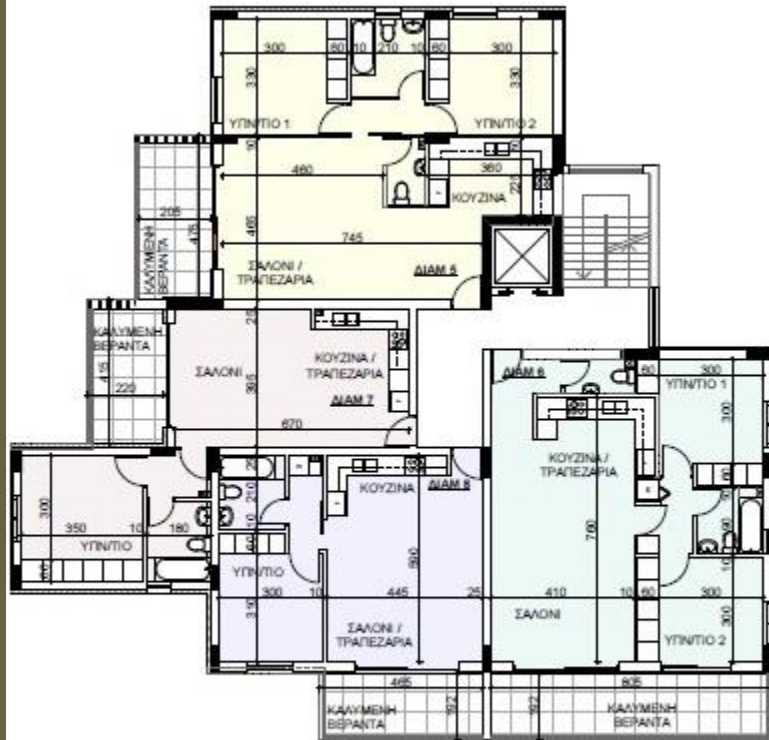
ΚΑΤΟΠΗ 'Α ΟΡΟΦΟΥ
