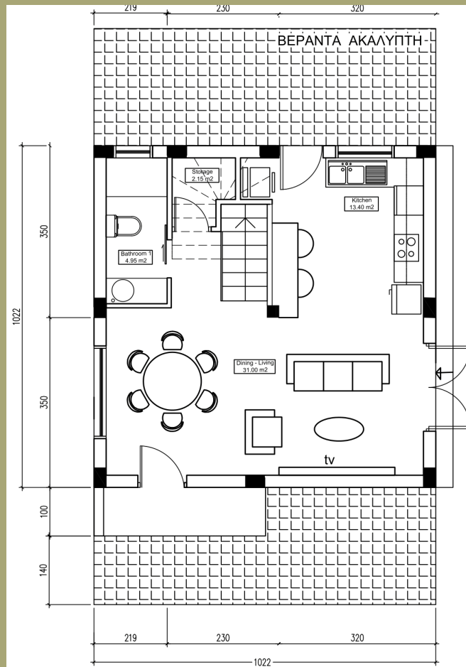
ΚΑΤΟΨΗ ΙΣΟΓΕΙΟΥ
