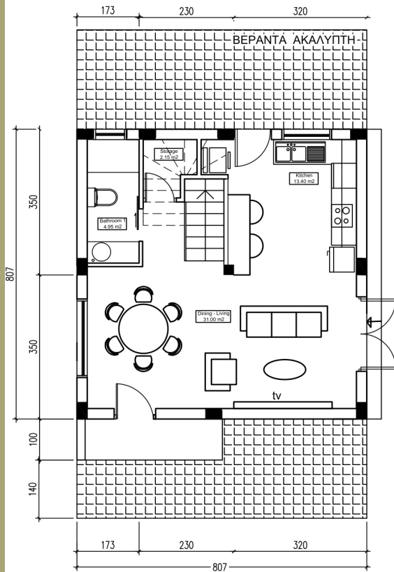
ΚΑΤΩΦΗ ΙΣΟΓΕΙΟΥ
