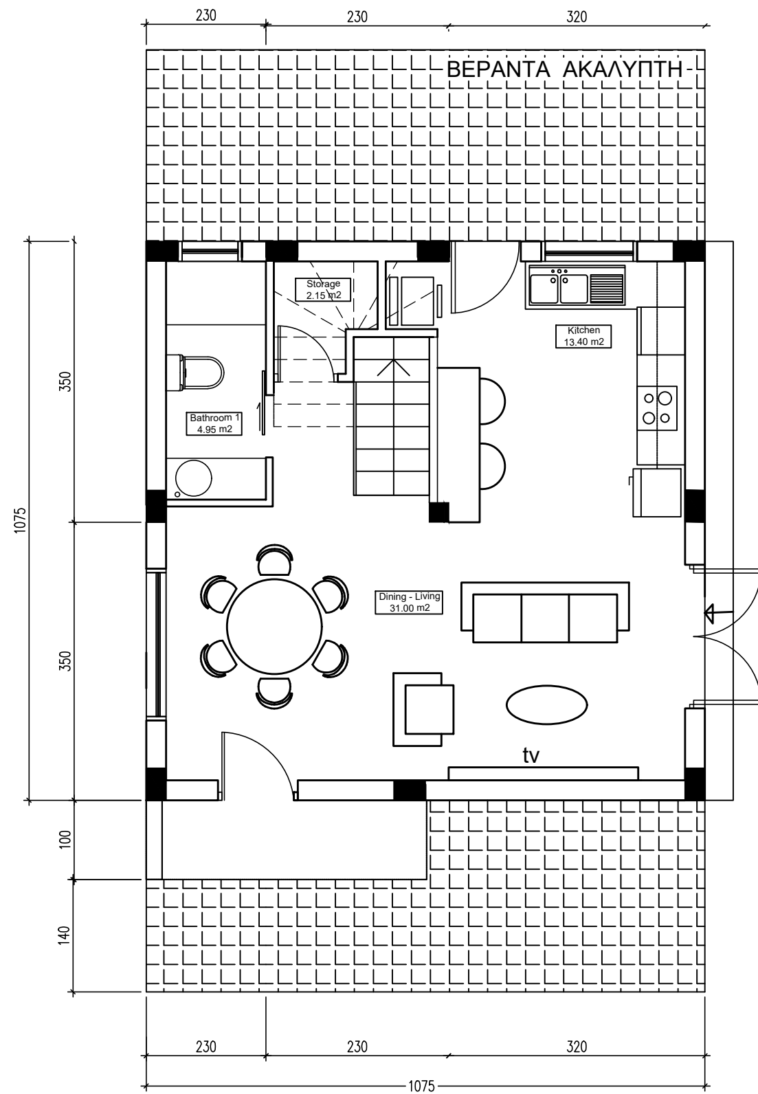
ΚΑΤΟΨΗ ΙΣΟΓΕΙΟΥ
