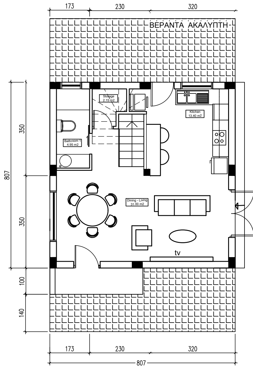
ΚΑΤΟΨΗ ΙΣΟΓΕΙΟΥ
